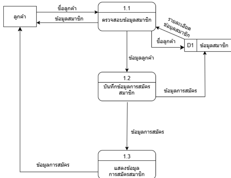
Data Flow Diagram (DFD) Level 2 Process การสมัครสมาชิก
