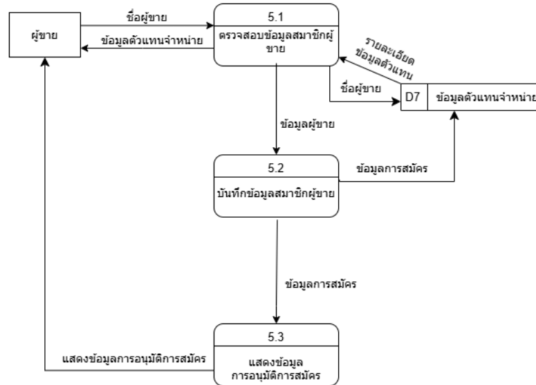
Data Flow Diagram (DFD) Level 2 Process การสมัครสมาชิกผู้ขาย
