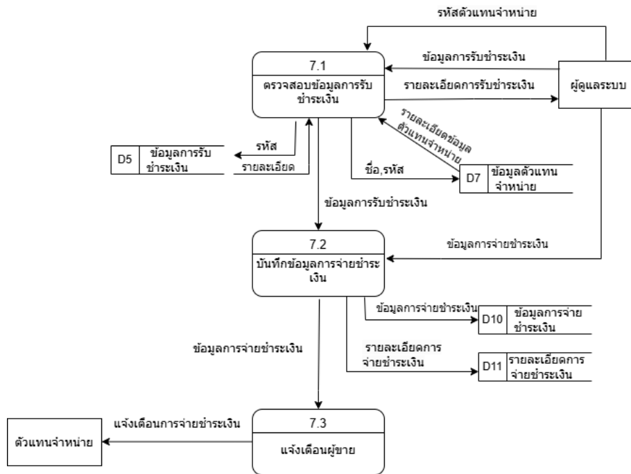
Data Flow Diagram (DFD) Level 2 Process การจ่ายชำระเงินให้ตัวแทนจำหน่าย
