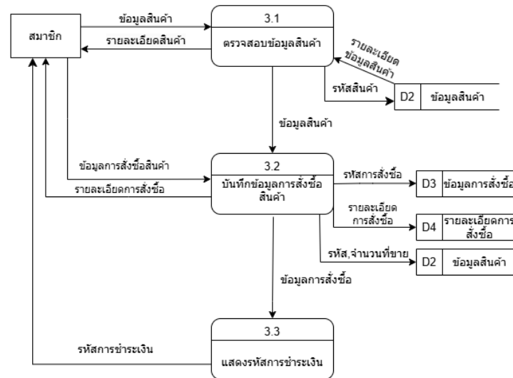
Data Flow Diagram (DFD) Level 2 Process การสั่งซื้อสินค้า
