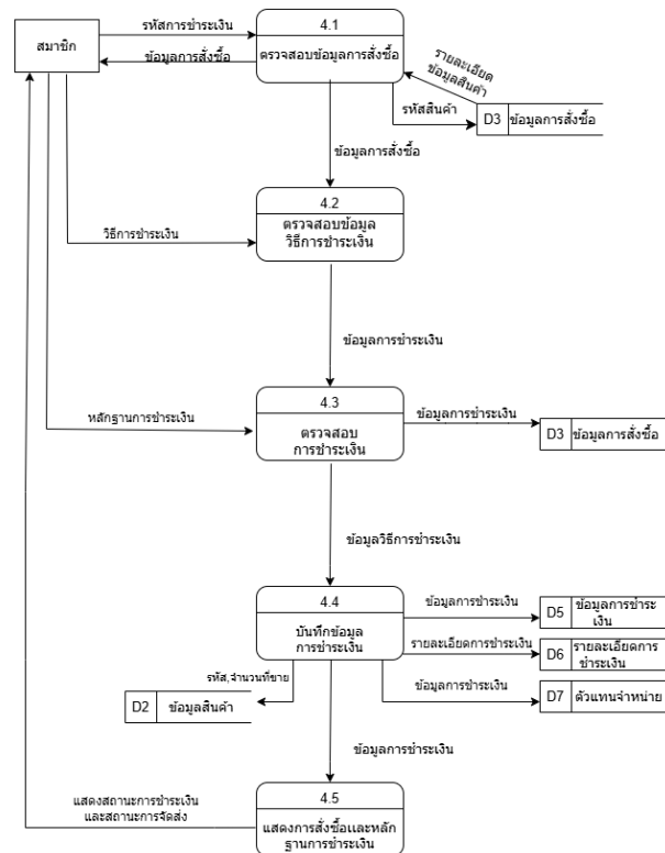
Data Flow Diagram (DFD) Level 2 Process การชำระเงิน
