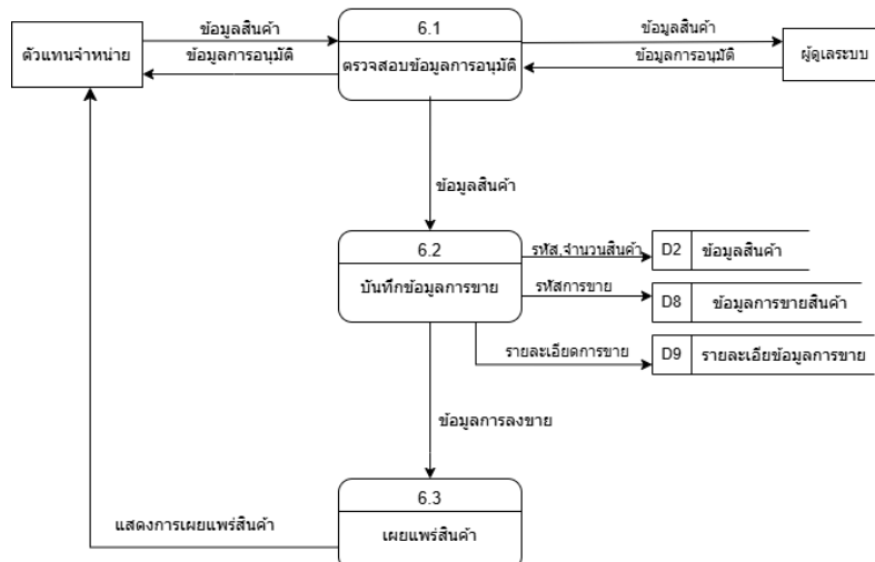
Data Flow Diagram (DFD) Level 2 Process การขายสินค้าสำหรับตัวแทนจำหน่าย
